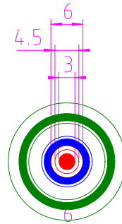
Achsmaße
