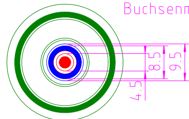
Radmaße
